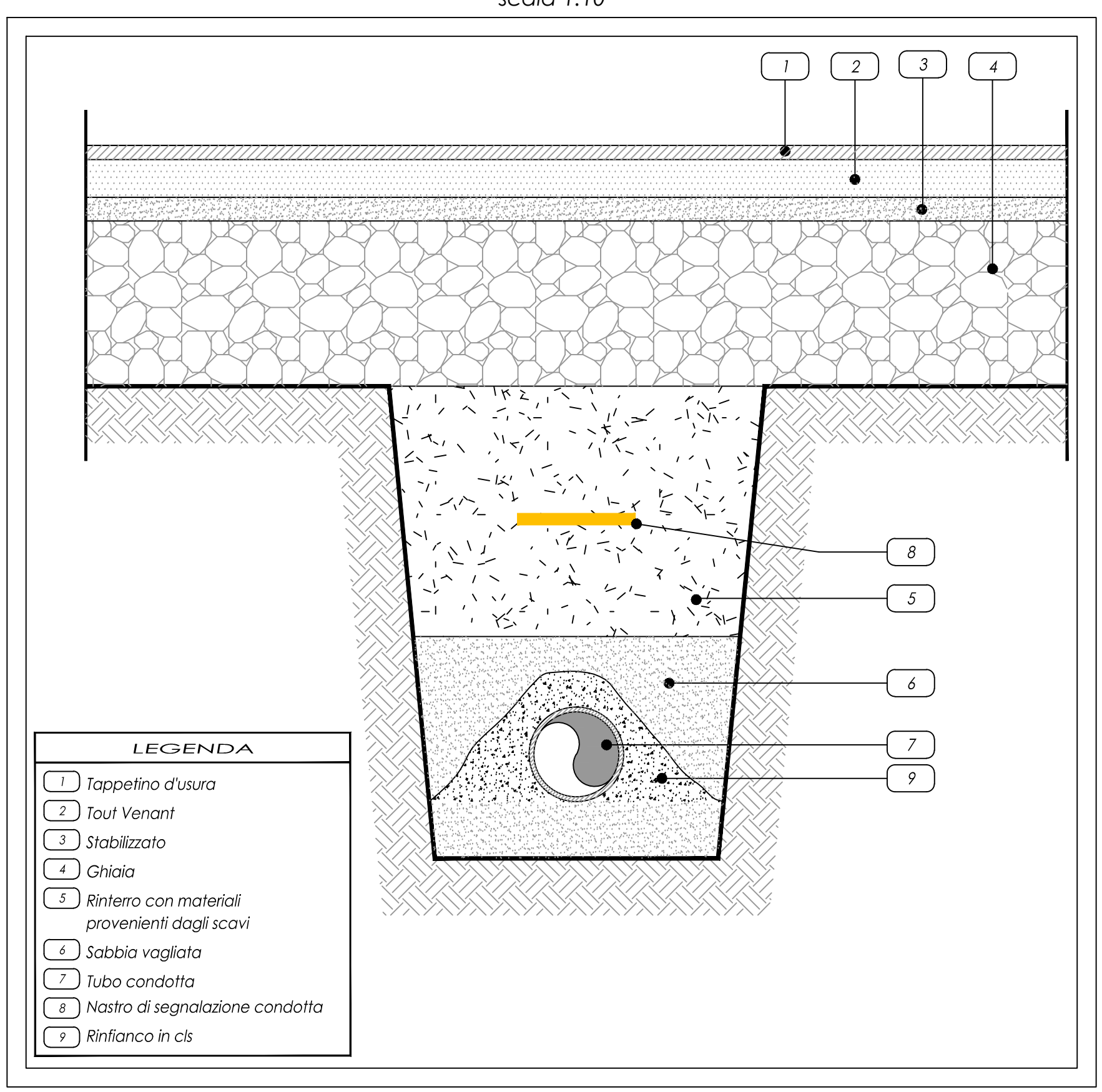
PARTICOLARE 2 SEZIONE DI SCAVO TIPO PER CONDOTTA INTERRATA scala 1:10
